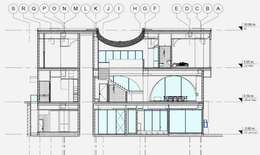
Sec A-A
