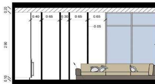
B4 4 نمای آشپزخانه Sc:1/5*
