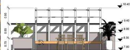
نما روبرو نشیمن Sc: 1/50
