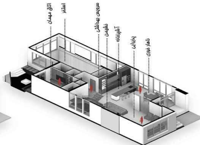
■ جانمایی فضاهای طبقه همکف
