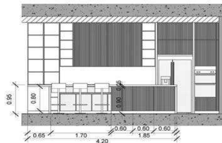
۴ نما روبرو میزبره آشپزخانه Sc: 1/50
