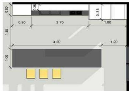
۱ پلان آشپزخانه همکف Sc: 1/50
