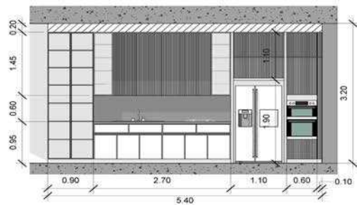
۲ نما روبرو کابینت آشپزخانه Sc: 1/50
