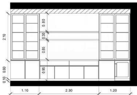
B4 3 نمای آشپزخانه Sc:1/5*
