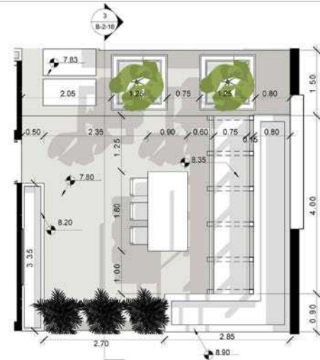
پلان اندازه گذاری و کد ارتفاعی Sc: 1/50
